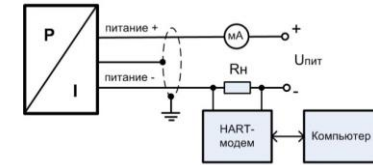
2-проводная линия (вых. сигнал - ток и HART)
