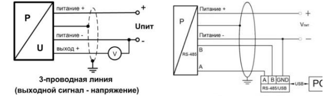
4-х проводная линия (интерфейс RS-485)
