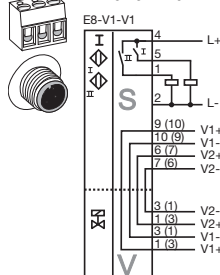
NBN3-F31K-E8-V1-V1 E8-V1-V1
