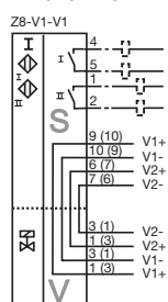
NBN3-F31K-Z8-V1-V1
