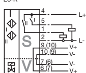
NBN3-F31K-E8-K E8-K
