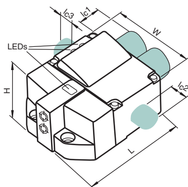
NBN3-F31K-E8
