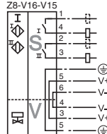
NBN3-F31-Z8-V16-V15
