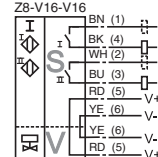
NBN3-F31-Z8-V16-V16
