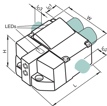
NBN3-F31K-Z8
